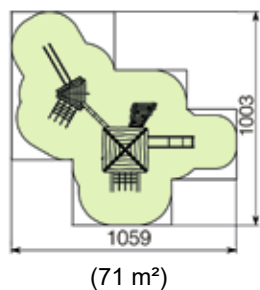
RO540 (combi-tovertoren met dak, met hanglussen) RO542 (combi-tovertoren met dak, met loopbalk)
